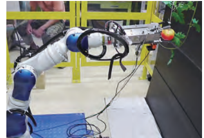
トマト収穫ロボットによる収穫実験
