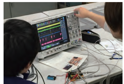
揺らぎ回路の特性試験
