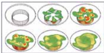
エンジンの燃焼解析
